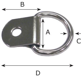
CLIP & DEE
